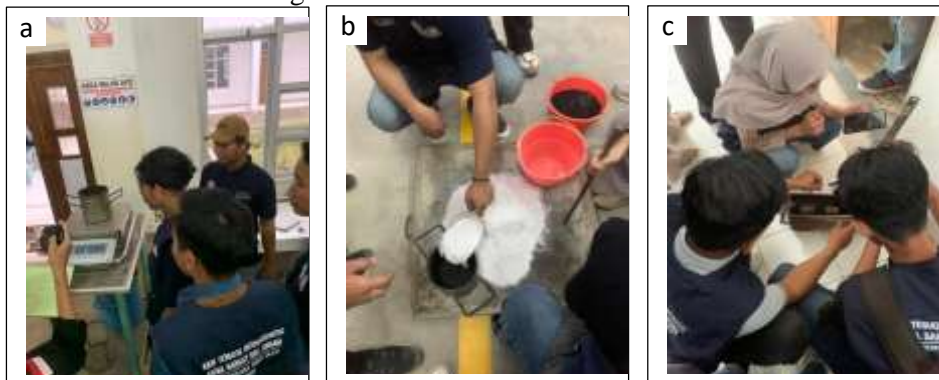
Gambar 4. Kegiatan mahasiswa KKN Tematik di laboratorium: (a) uji berat jenis material; (b) uji berat satuan bahan; (c) pengukuran volume cetakan batako
